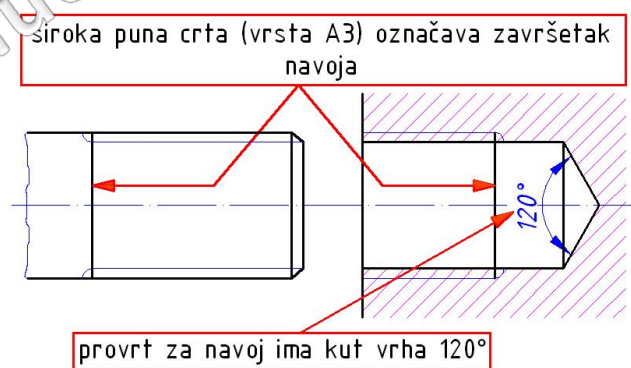
Slika 2. Završeci navoja
